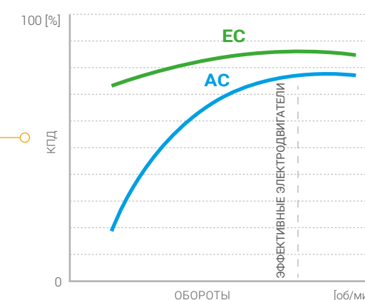
График зависимости КПД от скорости вращения
